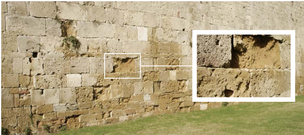
Opstijgend vocht > vernietigd oppervlak > zoutkristallen op het oppervlak
